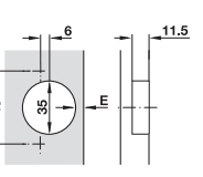
Drilling dimension ระยะเจาะ
