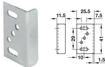
Angle striking plate เพลทรับกลอนแบบมุมฉาก
