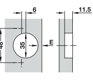
Drilling pattern ระยะเจาะ
