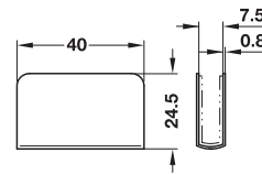
For timber door สำหรับบานไม้
