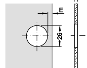
Drilling dimension ระยะเจาะ
