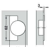
Cup dimension ขนาดถ้วยบานพับ
