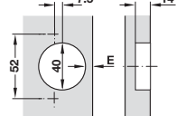
Drilling dimension ระยะเจาะ
