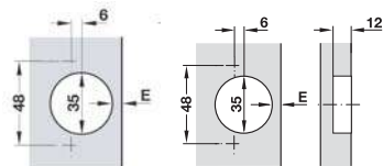
Cup dimension ขนาดถ้วยบานพับ
