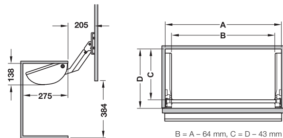
Picture shows installed fitting รูปแสดงการติดตั้งอุปกรณ์
