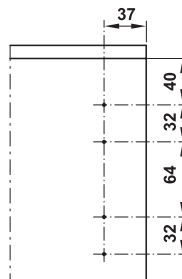
Drilling dimensions side panel ระยะที่แผงข้างตู้
