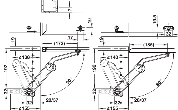
Flap with aluminium frame บานพร้อมโครงอลูมิเนียม
