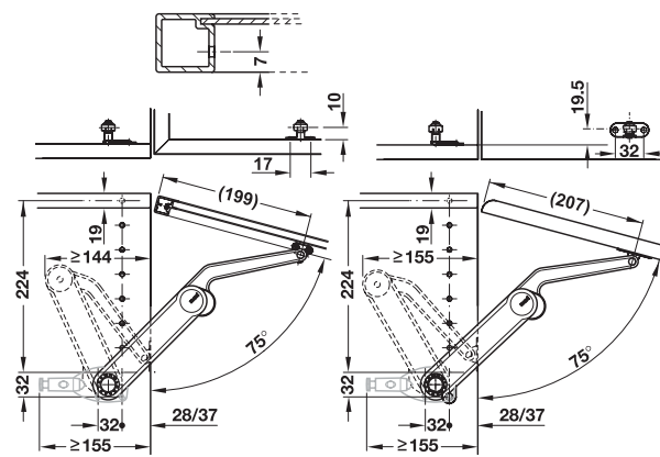
Flap with aluminium frame บานพร้อมโครงอลูมิเนียม
