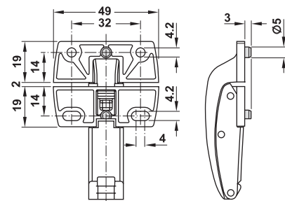
Mounting with chipboard screw and guide pin ติดตั้งโดยใช้สกรูเกลียวไม้ พร้อม โกดส์สลัก
