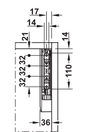
Drilling dimensions front panel ระยะเจาะที่หน้าบาน
