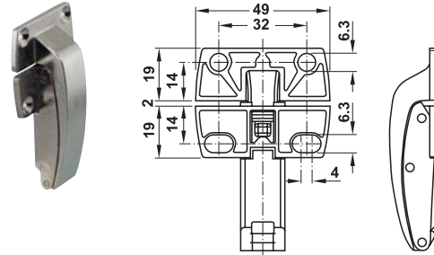
Mounting with VARIANTA special screw ติดตั้งโดยใช้สกรูแบบพิเศษ Varianta
