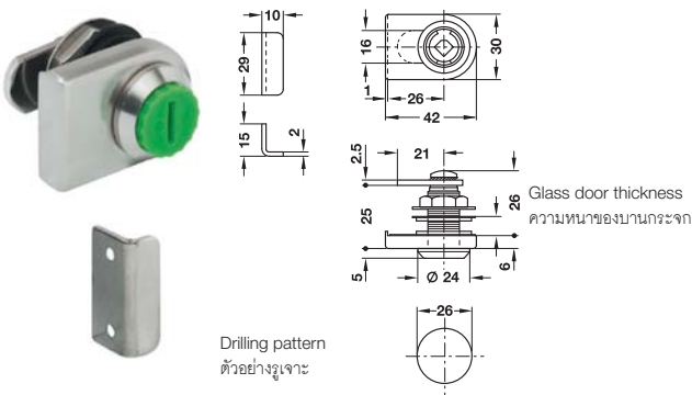
Installation การติดตั้ง
