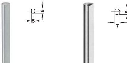
Profile rod Ø6 mm แกน Ø6 มม.
