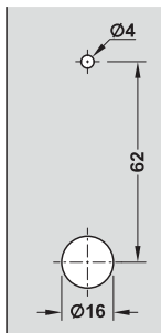
Drilling pattern รูปแบบการเจาะประตู
