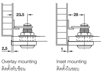
Installation การติดตั้ง
