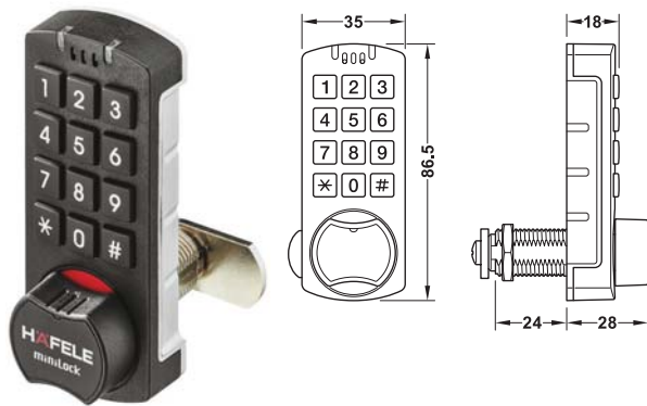
Locking cam ลิ้นล็อค
