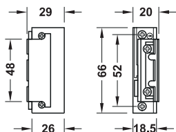
รหัสสินค้า 911.68.390: ไม่มีกลไกปลดล็อก
