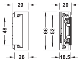
รหัสสินค้า 911.68.391: พร้อมกลไกปลดล็อก
