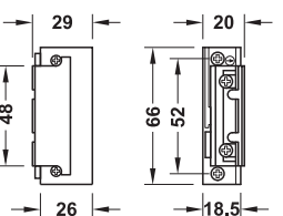
รหัสสินค้า 911.68.392: ไม่มีสวิตช์แสดงสถานะการทำงาน สามารถรับการจ่ายไฟฟ้าได้ตลอดเวลา
