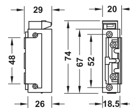
รหัสสินค้า 911.68.393: พร้อมสวิตช์แสดงสถานะการทำงาน สามารถรับการจ่ายไฟฟ้าได้ตลอดเวลา
