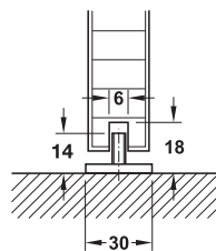
Floor guide without guide track in door leaf การติดตั้งกันแกว่งแบบไม่มีรางล่าง
