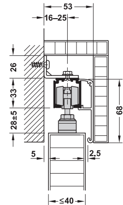
Wall mounting with mounting bracket and fixing clip for wooden panel การติดตั้งบนผนังด้วยเพลาติดตั้งผนังและฝาปิดแบบคลิปสำหรับบานไม้
