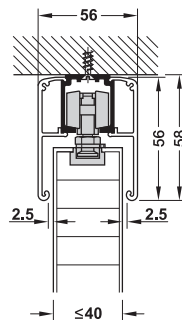
Ceiling installation with running track mounting bracket and wide clip panel 56 mm การติดตั้งบนเพดานพร้อมฝาครอบแบบคลิป 56 มม.
